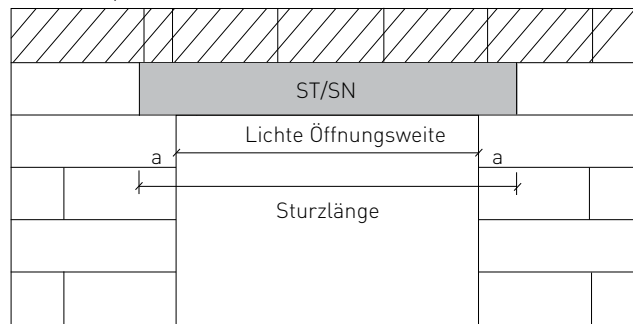
a) Auflagertiefe
