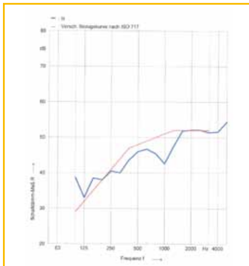
Schalldämm-Maß von 20 cm YTONG Multipor auf einer 24 cm dicken Wand aus YTONG Verbundsteinen (P4/0,60).
